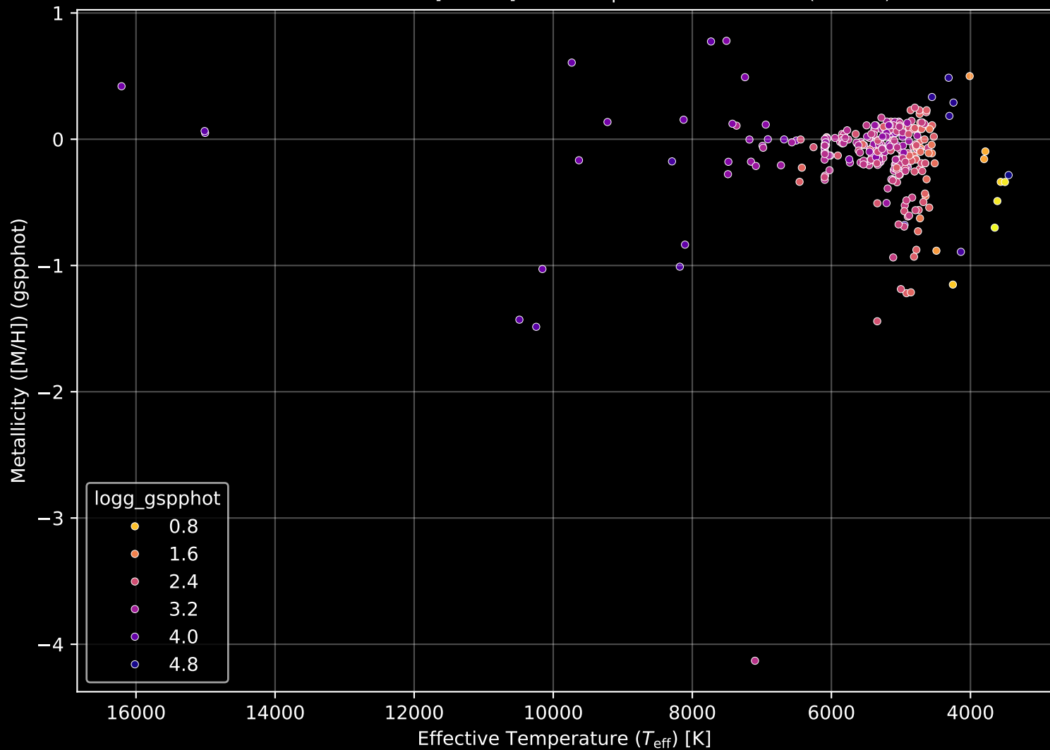
APOGEE DR17 Field: [240-04] Stellar Population Parameters (n= 317)
